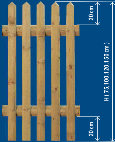
Halbrundriegel für Senkrecht- und Scherenzaun unterschiedliche Längen und Breiten
