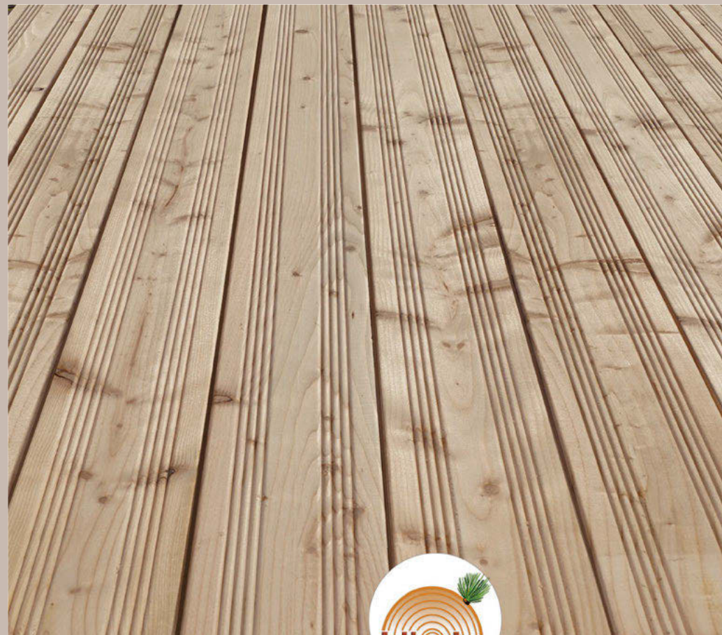
Bodendiele aus Lärche 2,0 cm stark, 12,0 cm breit, roh, beide Breitseiten fein geriffelt.
