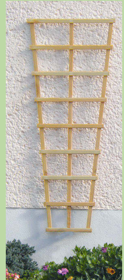
Rankgitter Rhodos Stäbe 1,2 x 3,0 cm, gehobelt, kesseldruckimprägniert
